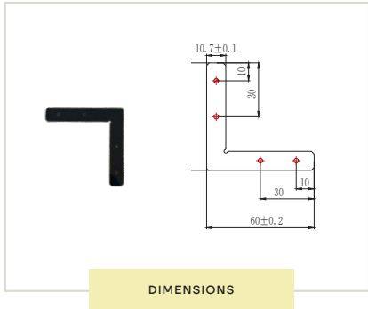
Mini Hybrid L Bracket
