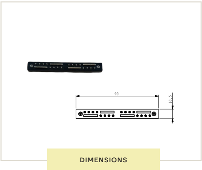
Mini Hybrid I Joint
