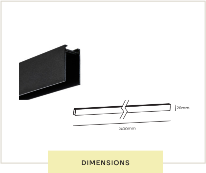
Mini Hybrid 2.4M Profile A
