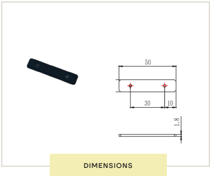
Mini Hybrid Straight Bracket
