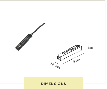
Mini Hybrid End Feeder
